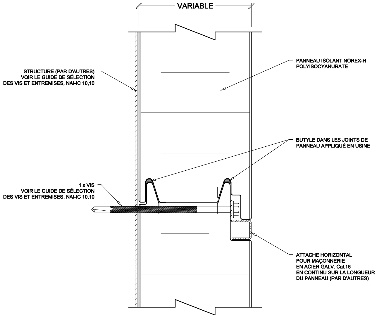
VUE DE LA SECTION AUX ENTREMISES
